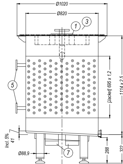
Seitenansicht
